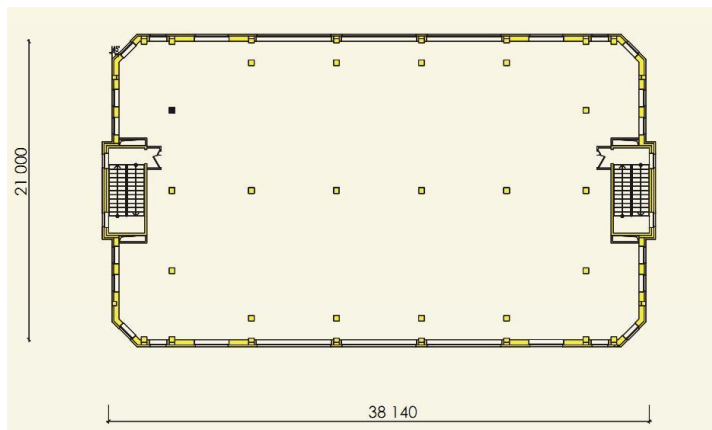
3 этаж
