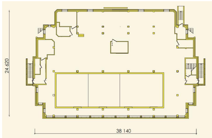
3 этаж
